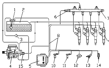
Рис. 5.1. Схема топливной системы: 1 -фильтр-топливоприемник; 2 -топливный бак; 3 -подкачивающий насос с топливным фильтром в сборе; 4 -ТНВД; 5 -электронный блок управления (ЭБУ); 6 -датчик давления топлива в аккумуляторе; 7 -аккумулятор топлива (рампа); 8 -жгут проводов; 9 -форсунка; 10 -датчик частоты вращения распредвала; 11 -датчик частоты вращения коленвала; 12 -датчик положения педали акселератора; 13 -датчик давления наддува; 14 -датчик температуры охлаждающей жидкости; 15 -электромагнитный клапан остановки двигателя
