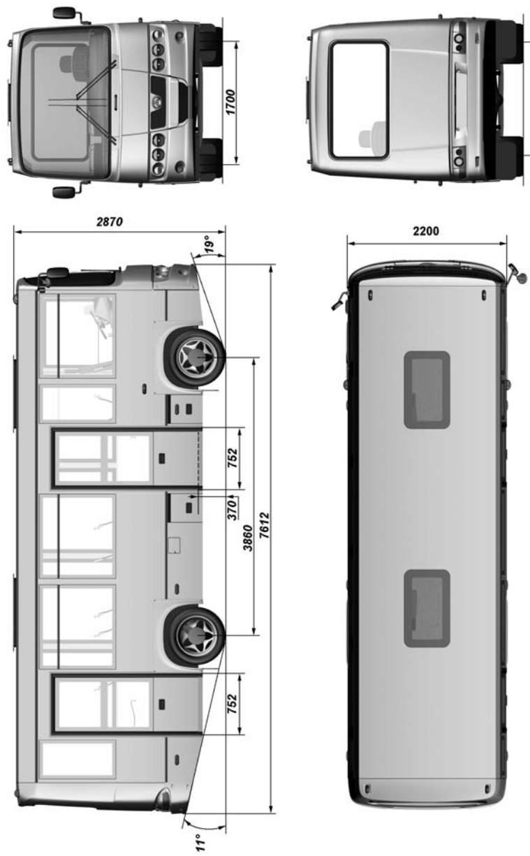
Рис. 1.1. Габаритные размеры автобуса 2245 (размеры даны для справок)
