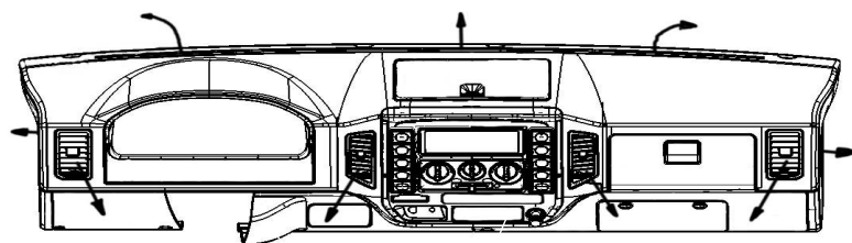
Рис. 3.13 Распределение воздушных потоков в кабине
