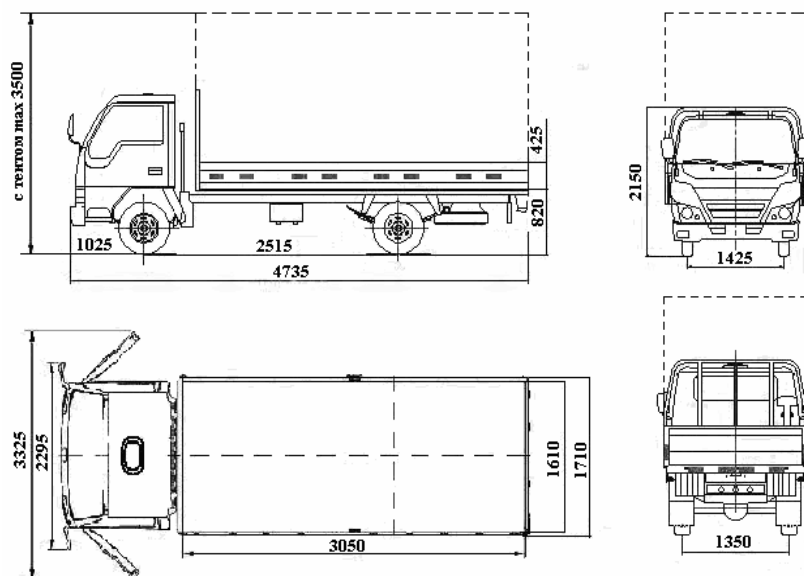
Рисунок 1.5 Автомобиль ВАУ Фених 33463-0000010
